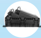
Cierre de empalme QuickNap para 8 acopladores SC simplex y 36 empalmes
